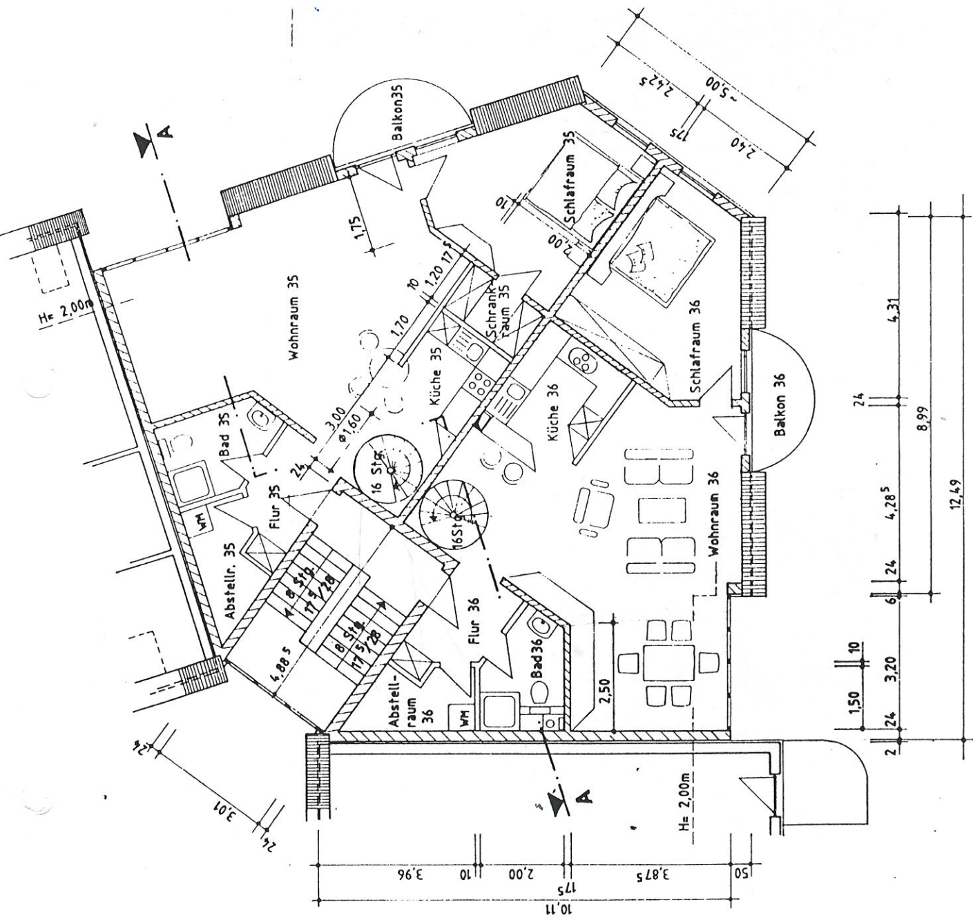
Grundriß Dachgeschoß Gebäude 4
