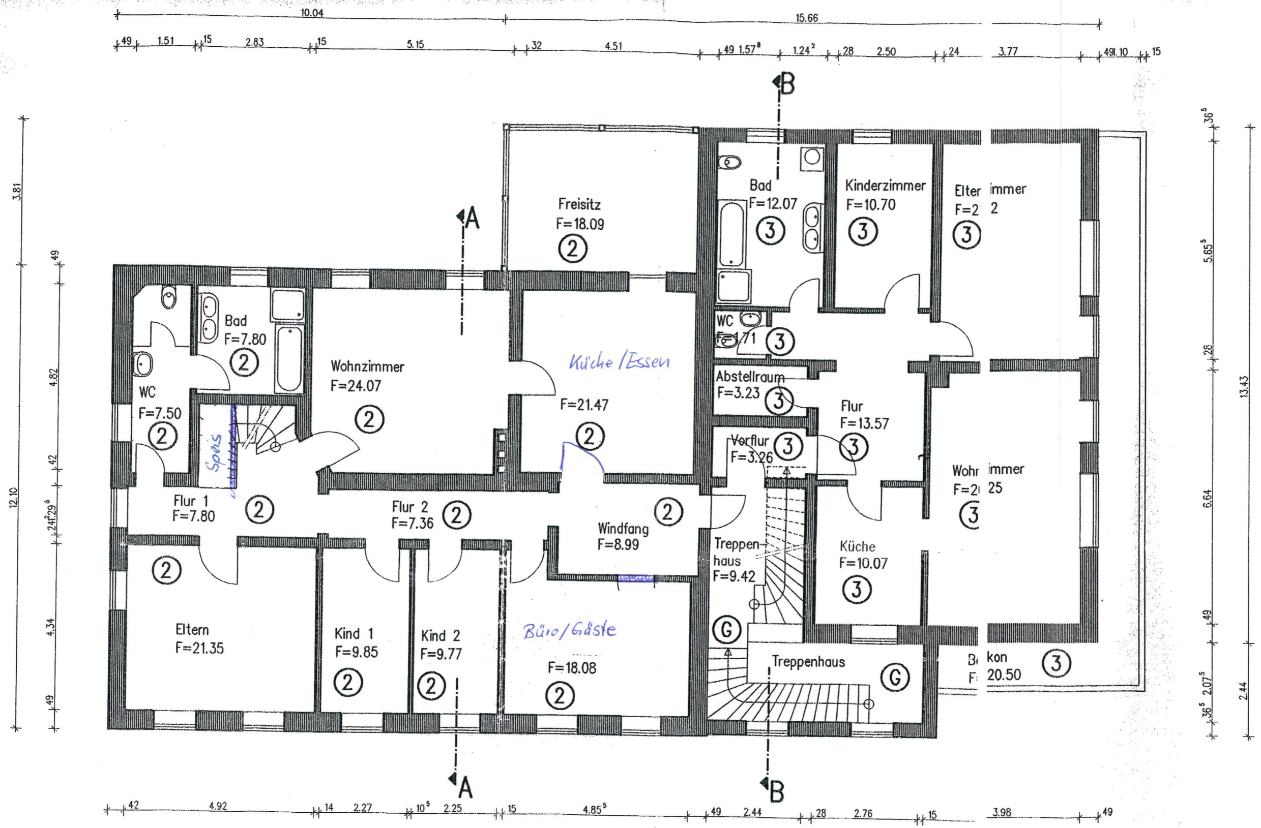
Obergeschoss
